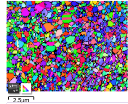
加工と熱処理による組織(結晶粒)の微細化
