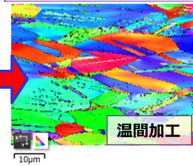
冷間加工、温間加工の組織の違い
