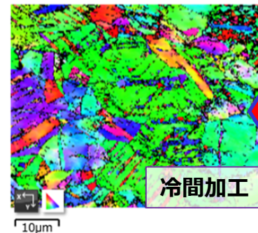
冷間加工、温間加工の組織の違い
