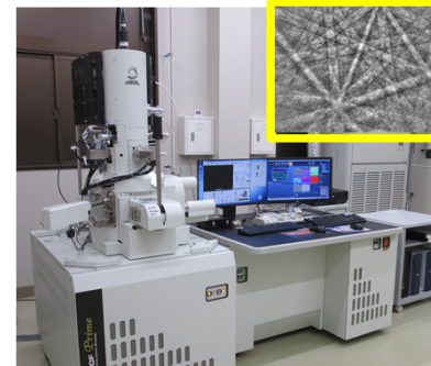
FE-SEM/EDS/EBSD
