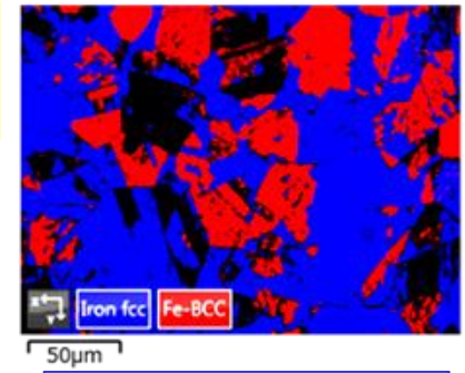
2相材料の結晶相マップ
