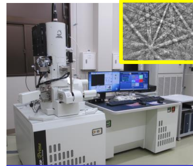
FE-SEM/EDS/EBSD
