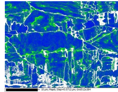
局所方位差による ひずみマップ
