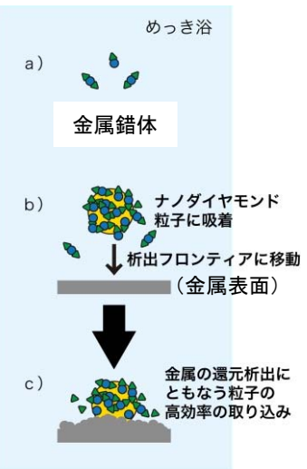
ナダイヤモンドの共析メカニズム(推定)
