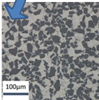
MMCのマイクロ組織
