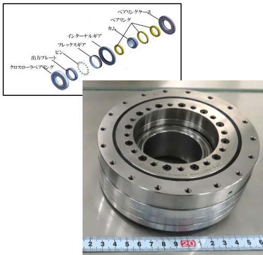
新方式波動歯車減速機 (特許出願済)
